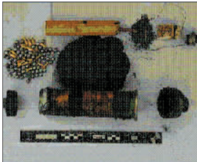
阿不都热西提·阿不来提、依明·色买尔制作的爆炸装置及其结构拆解图。
