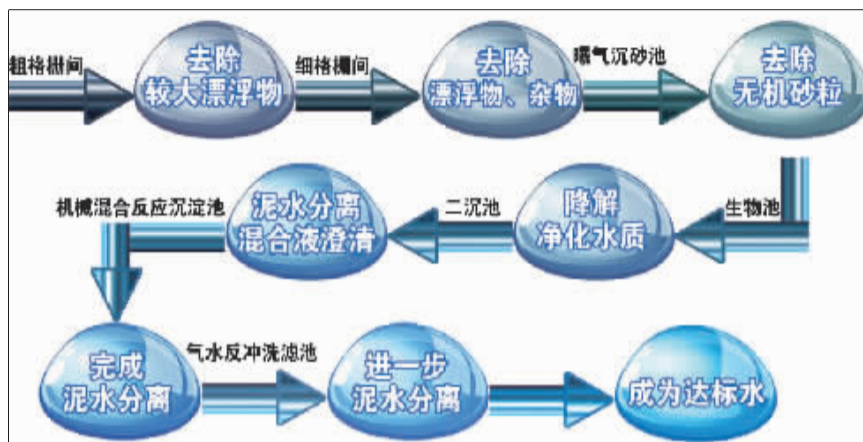
污水处理过程示意图
