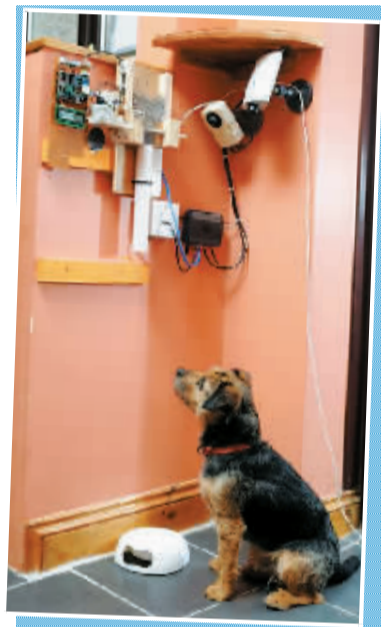
自动喂食机
