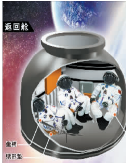
神舟九号返回舱结构示意图 (新华社发)
