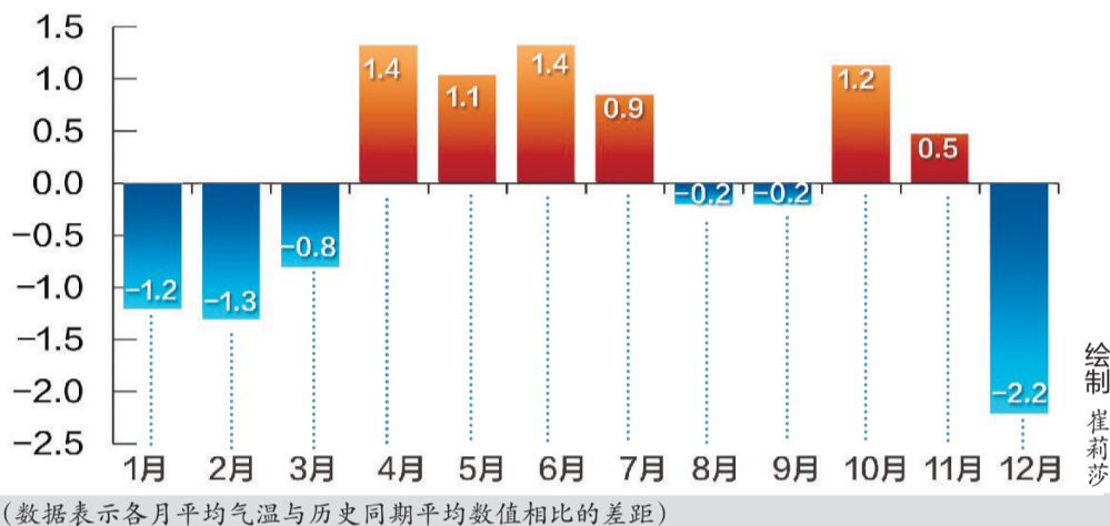
全市2012年各月平均气温距平图(单位:℃)
