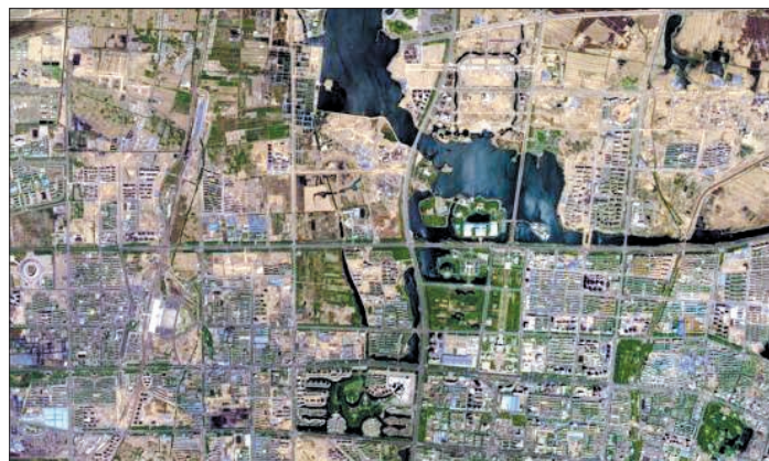
“高分一号”卫星银川影像
