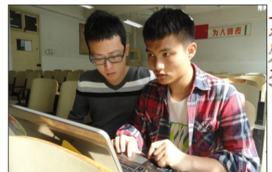
王元成(右)
