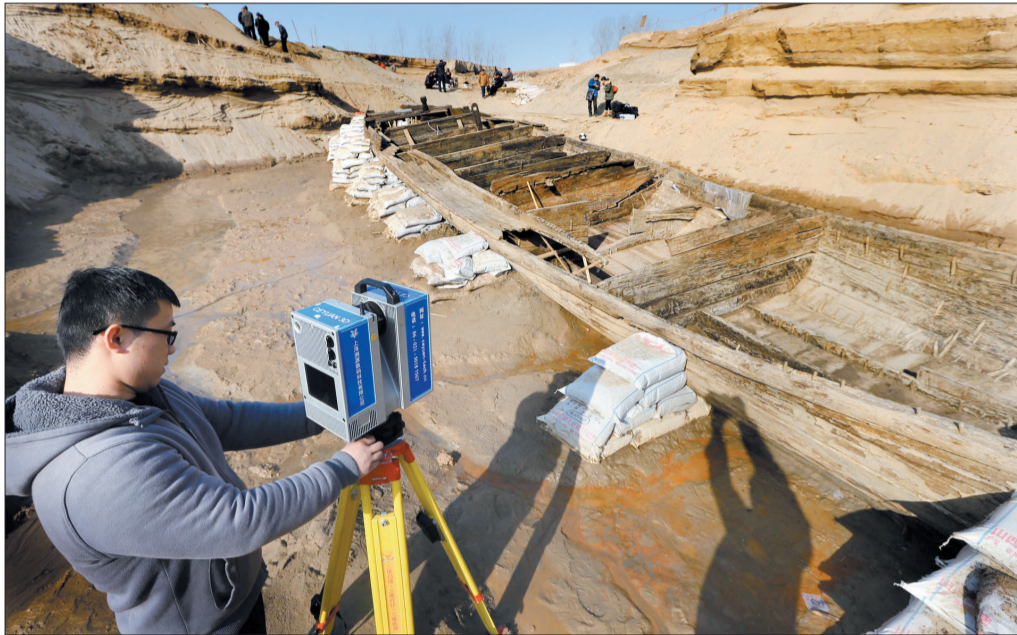
激光扫描仪在录入数据
