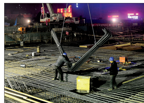
深夜,吊装钢筋骨架工作区灯火通明
