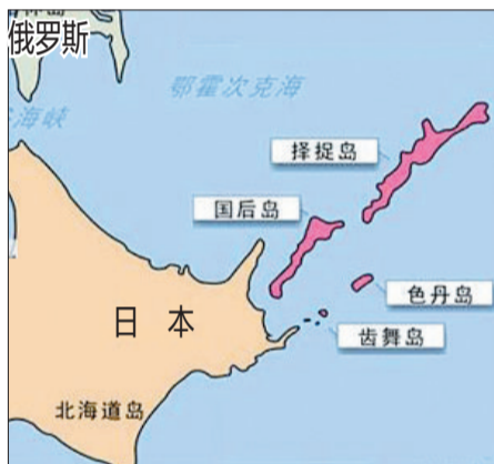
千岛群岛示意图
