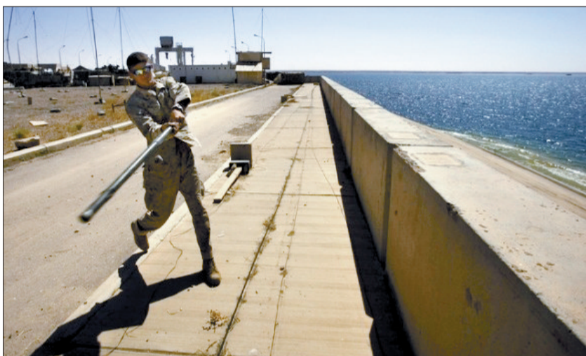
2005年,一名驻防伊拉克哈迪萨大坝的美军士兵在大坝上击打石块(网络图片)
