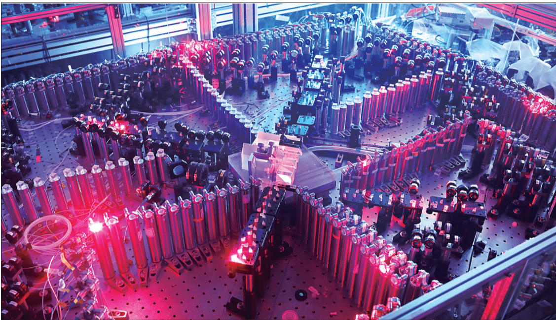
这是光量子干涉实物图：左下方为输入光学部分，右下方为锁相光路，上方共输出100个光学模式，分别通过低损耗单模光纤与100超导单光子探测器连接 (新华社发)
